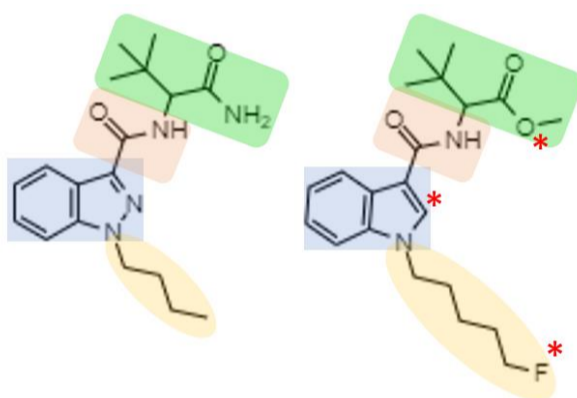
Mynd 2. Efnafræðileg samsetning ADB-BUTINACA og 5F-MDMB-PICA. Rauð stjarna sýnir efnafræðilegan mun á milli efnanna. Lituðu svæðin sýna svo kjarna, tengil, tengihóp og hala.
